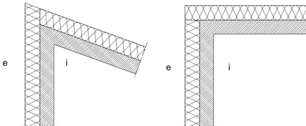
Abbildung 3.5 Darstellung einer spitz zulaufenden Außenecke (links) und einer optimierten Ausführung (rechts)
