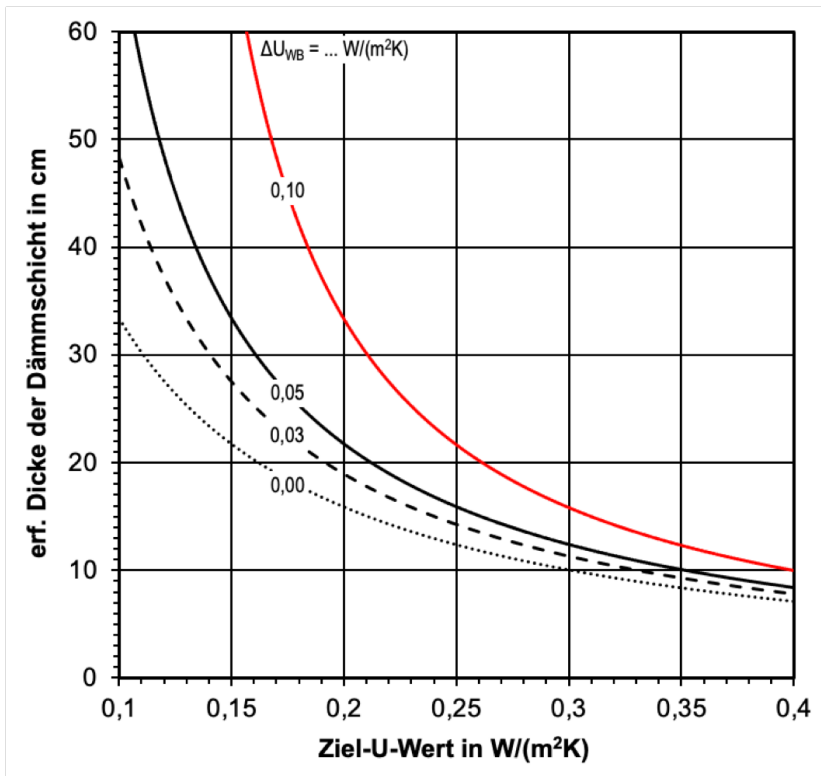
Abbildung 3.3 Beeinflussung der erforderlichen Dämmschichtdicken durch den Wärmebrückenzuschlag \Delta U_{WB}
