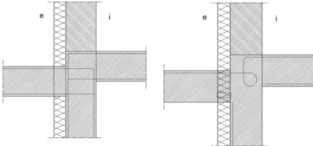
Abbildung 3.6 Darstellung einer nicht entkoppelten Durchdringung der Dämmebene im Bereich einer Balkonplatte (links) und des optimierten thermisch getrennten Anschlusses (rechts)
