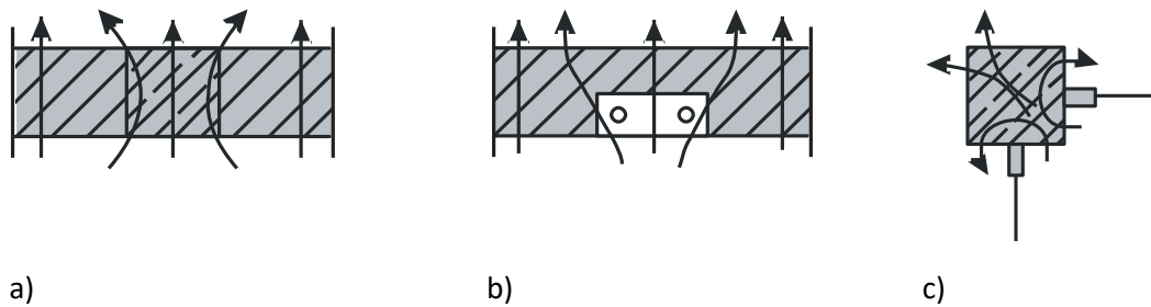
Abbildung 3.1 Beispiele für Wärmebrücken
