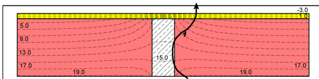
Abbildung 3.2 Verlauf von Isothermen und Wärmestrom
